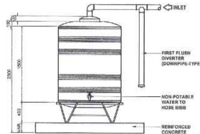
LEFT-SIDE ELEVATION
