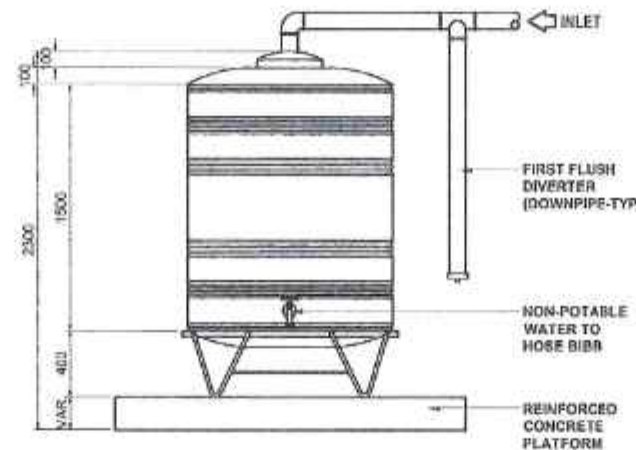
LEFT-SIDE ELEVATION
