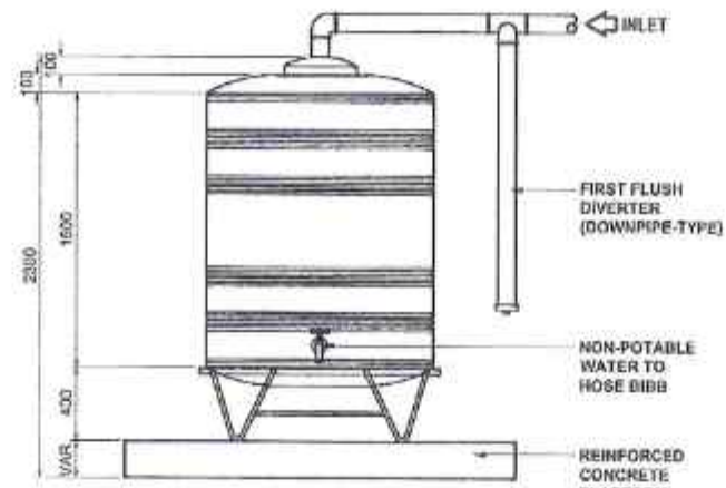
LEFT-SIDE ELEVATION
