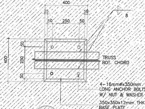
9A PLAN S-18 SCALE 1:10 M.
