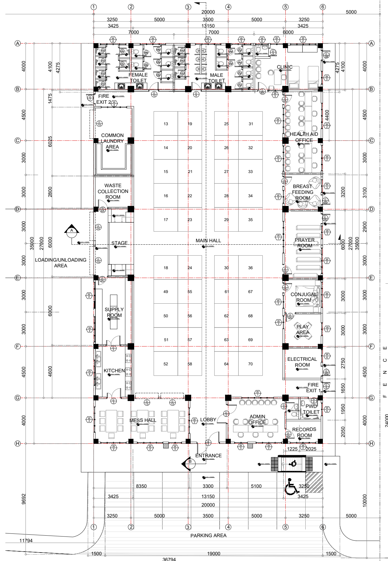
1 FLOOR PLAN A 2 SCALE: 1:200M
