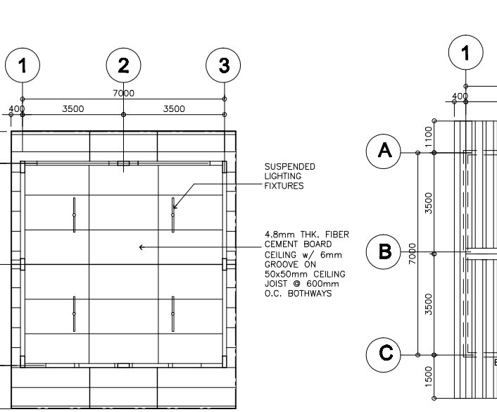
8 REFLECTED CEILING PLAN A-2 SCALE: 1:100M
