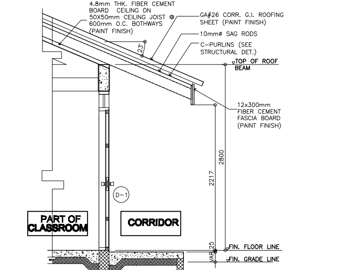
13 VENT. DET. PLAN A-2 SCALE: 1:20M
