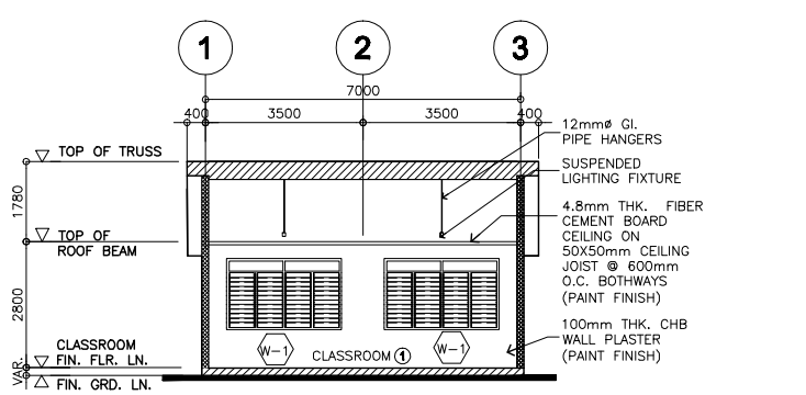
7 LONGITUDINAL SECTION A-2 SCALE: 1:100M
