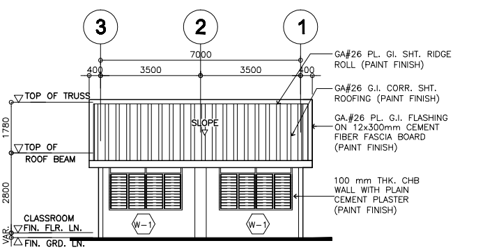
5 REAR ELEVATION A-2 SCALE: 1:100M
