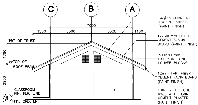
3 RIGHT ELEVATION A-2 SCALE: 1:100M
