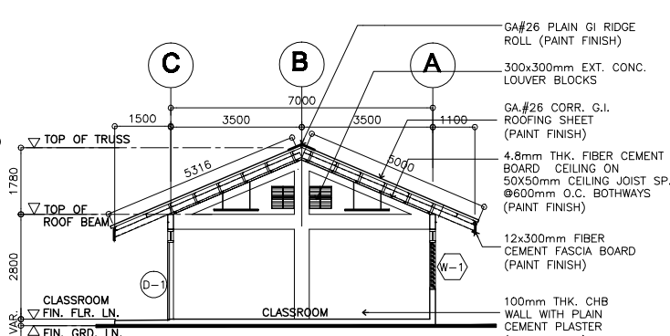
6 CROSS SECTION A-2 SCALE: 1:100M
