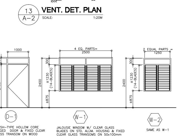
15 SCHEDULE OF DOORS & WINDOWS A-2 SCALE: 1:100M
