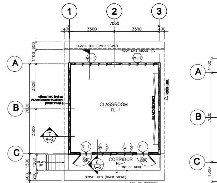
1 FLOOR PLAN A-2 SCALE: 1:100M
