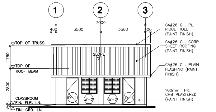
2 FRONT ELEVATION A-2 SCALE: 1:100M
