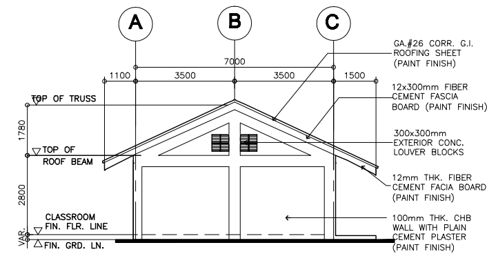
4 LEFT ELEVATION A-2 SCALE: 1:100M
