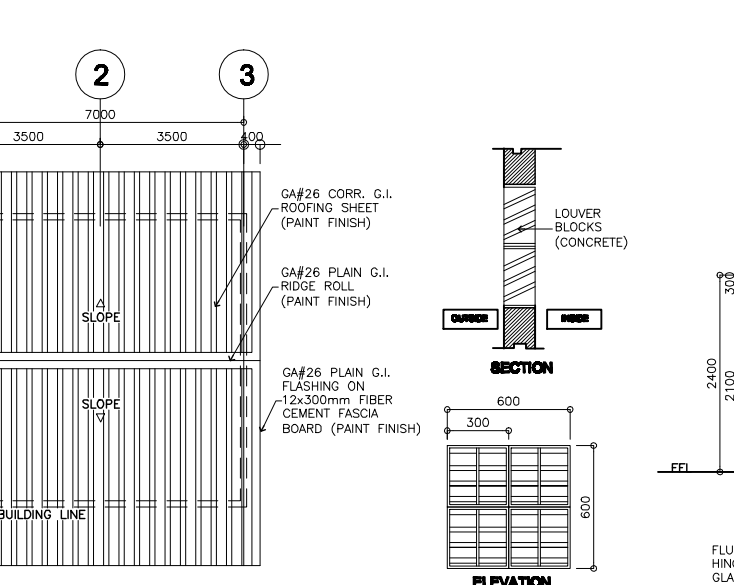
9 ROOF PLAN A-2 SCALE: 1:100M
