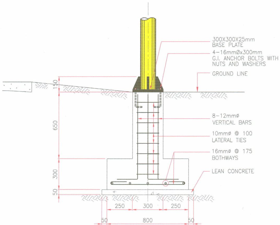
ELEVATION
